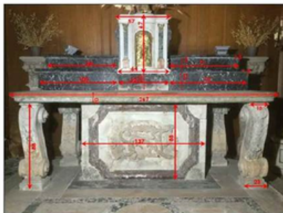
ELEVATION OCCIDENTALE
